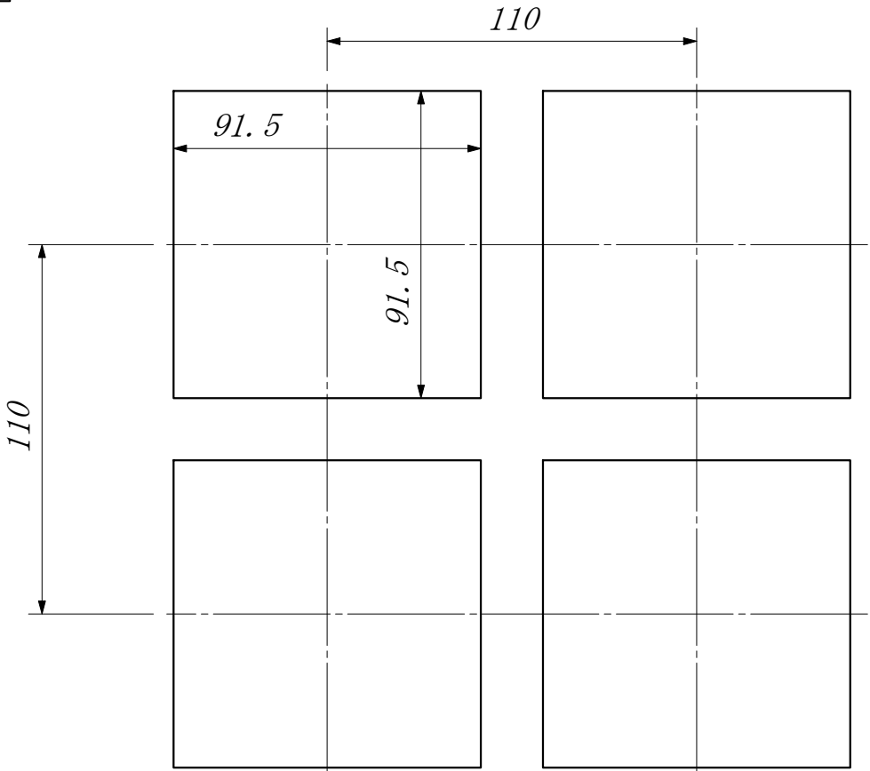
パネルカット (縮尺1/2)
